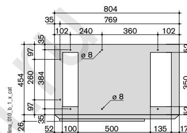
Plan de découpe C
