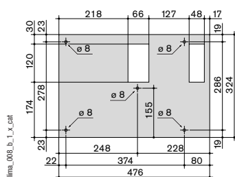
Plan de découpe A
