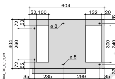
Plan de découpe B
