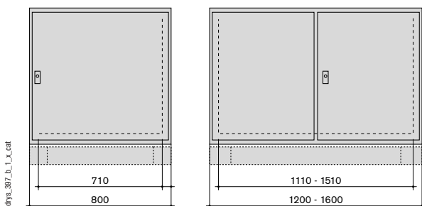
Coffret AE
